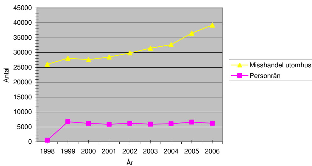
Diagram 3: Polisanmälda misshandelsbrott (utomhus) och personrån i Sverige 1998-2006
