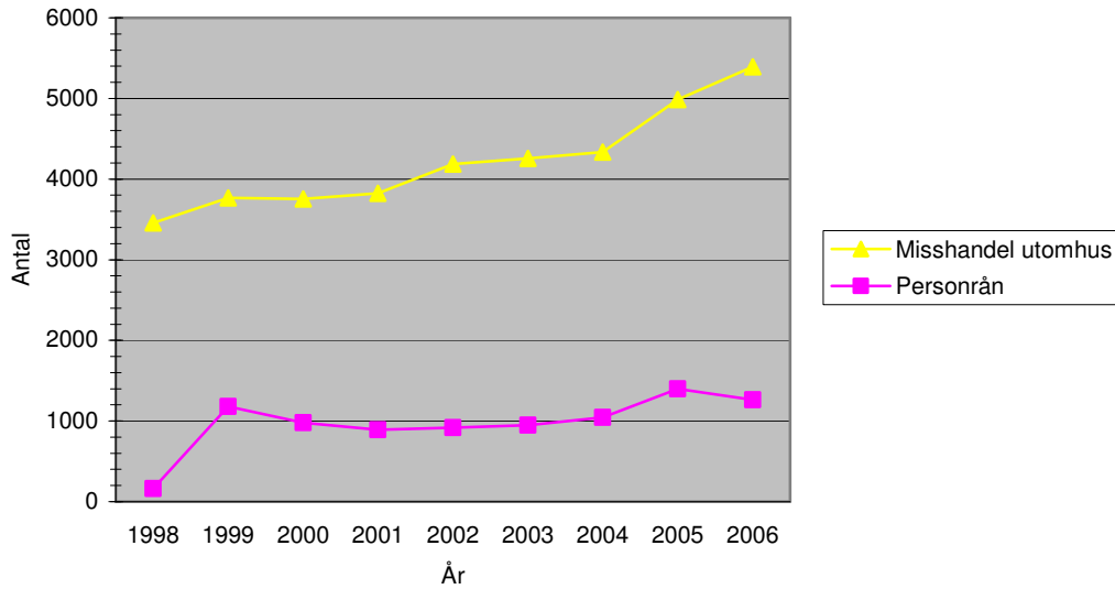
Diagram 2: Polisanmälda misshandelsbrott (utomhus) och personrån i Skåne län 1998-2006
